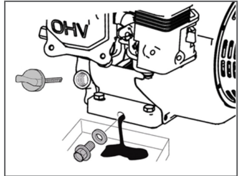
Рис. 16 Замена моторного масла
