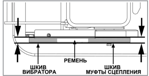
Рис. 24 Проверка натяжения ремня привода вибратора
