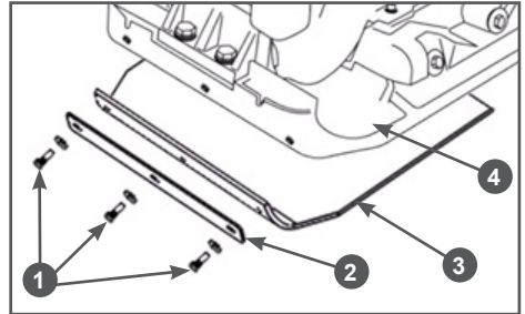
Рис. 3 Установка резинового коврика
