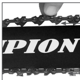
Рис.8 Правильное натяжение цепи
