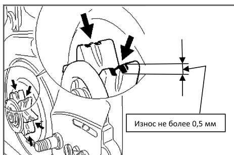
Рис.10 Проверка износа звездочки
