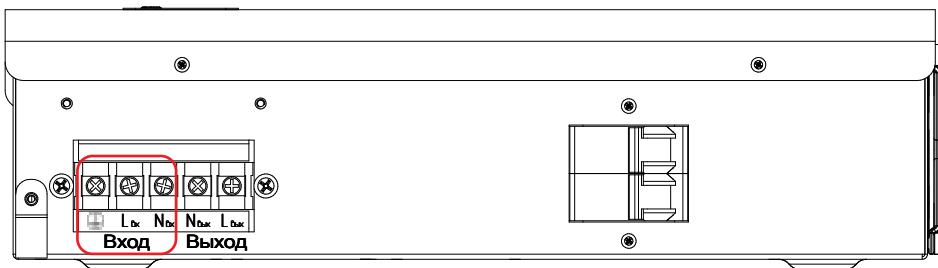
Рисунок 26. Стабилизатор Штиль IS5000. Выводы «Вход» — L-N»
