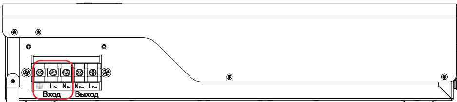
Рисунок 27. Стабилизатор Штиль IS7000. Выводы «Вход» — L-N»
