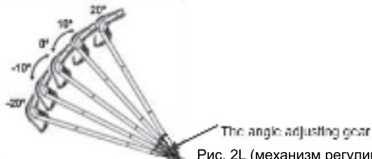
Рис. 2L (механизм регулировки угла наклона)
